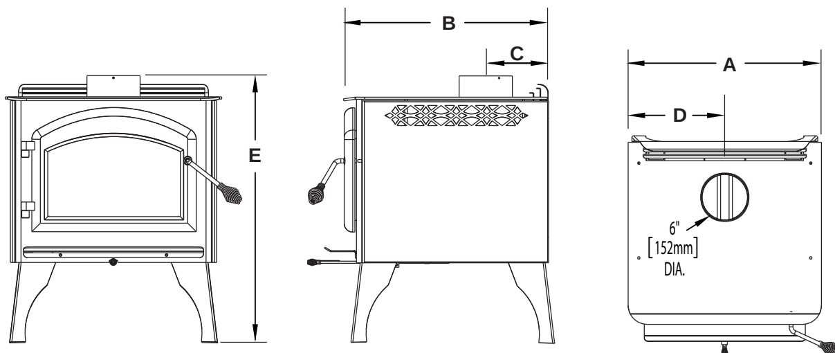
1400PL ILLUSTRÉ
