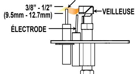
LA FLAMME DOIT ENVELOPPER LA PARTIE SUPÉRIEURE DE LA SONDE DE FLAMME DE 3/8\" (9.5mm) À 1/2\" (12.7mm)
